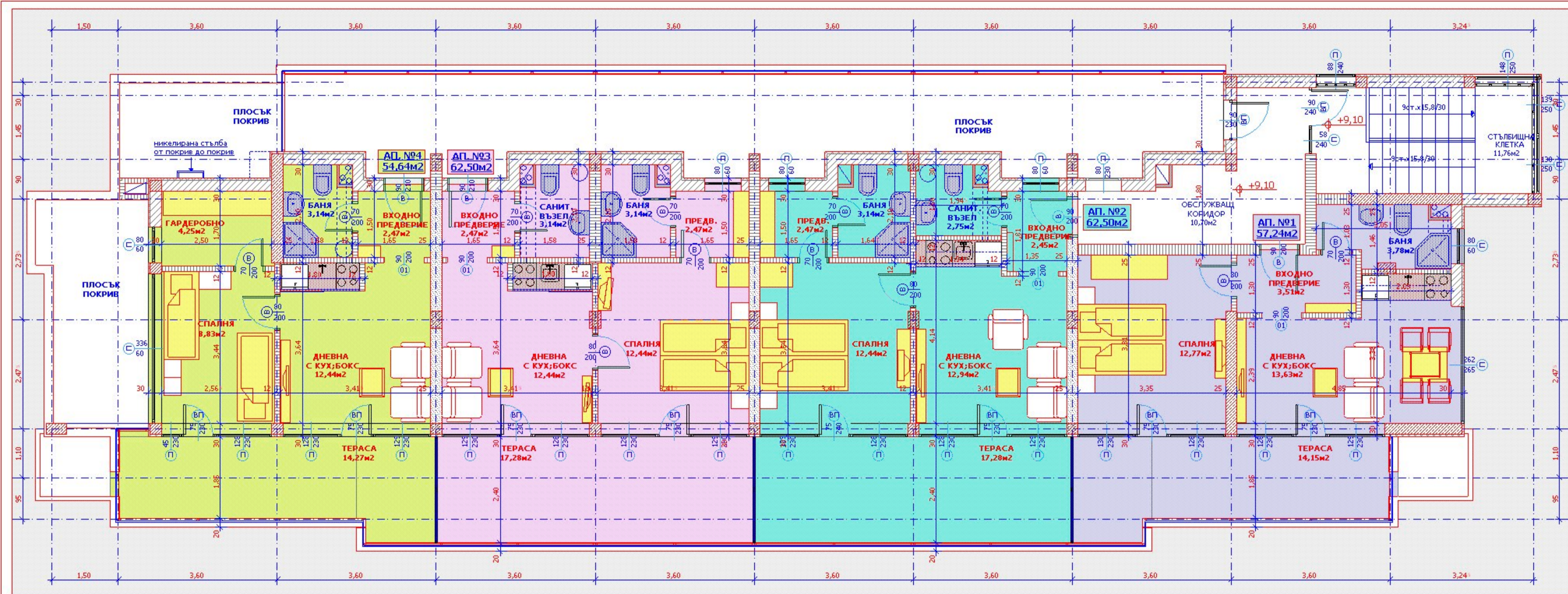
РАЗПРЕДЕЛЕНИЕ НА ТАВАНСКИ ЕТАЖ "КОТА +9.10" М 1:50
