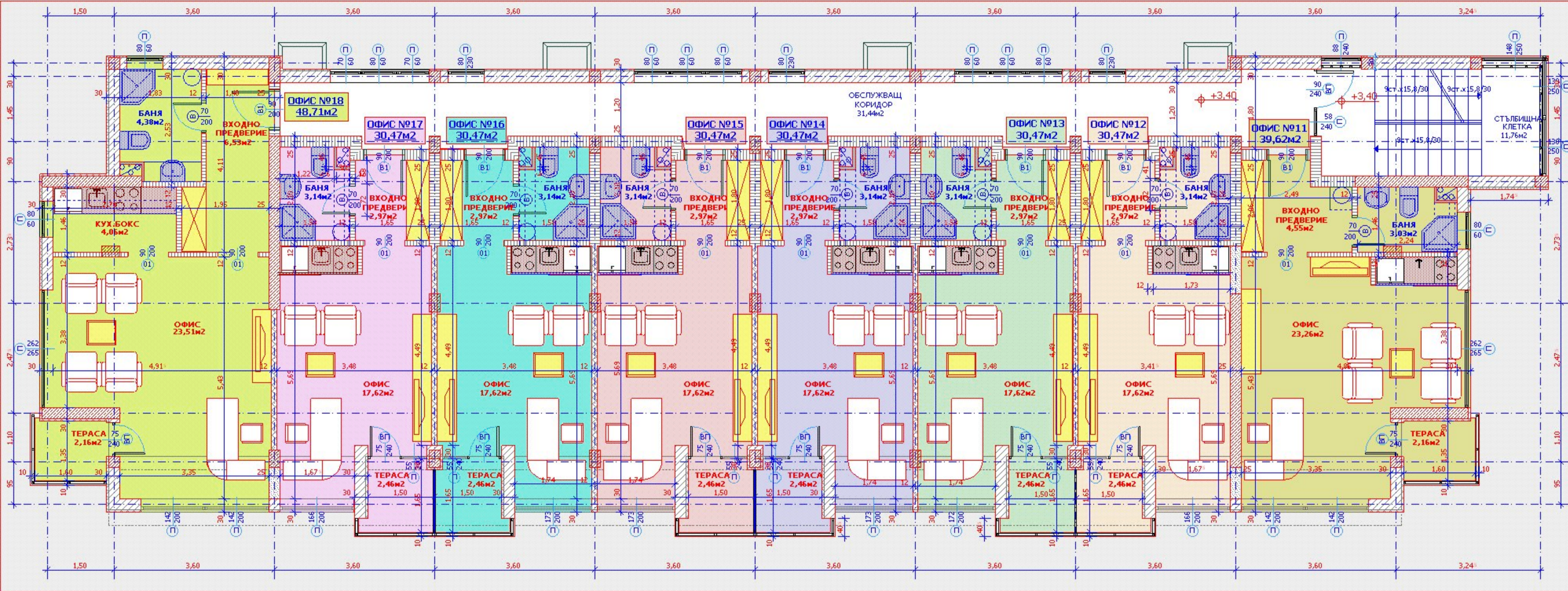
РАЗПРЕДЕЛЕНИЕ НА ВТОРИ ЕТАЖ "КОТА +3,40" М 1:50
