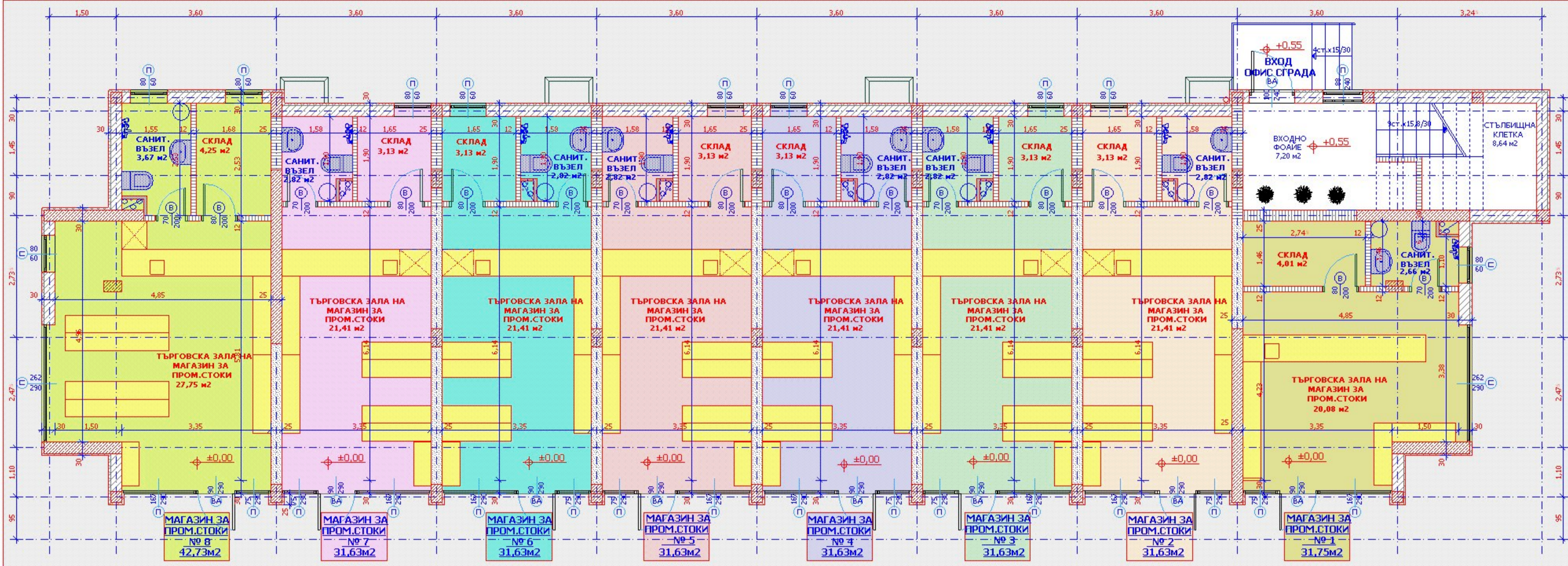
РАЗПРЕДЕЛЕНИЕ НА ПЪРВИ ЕТАЖ "КОТА +/-0.00" М 1:50
